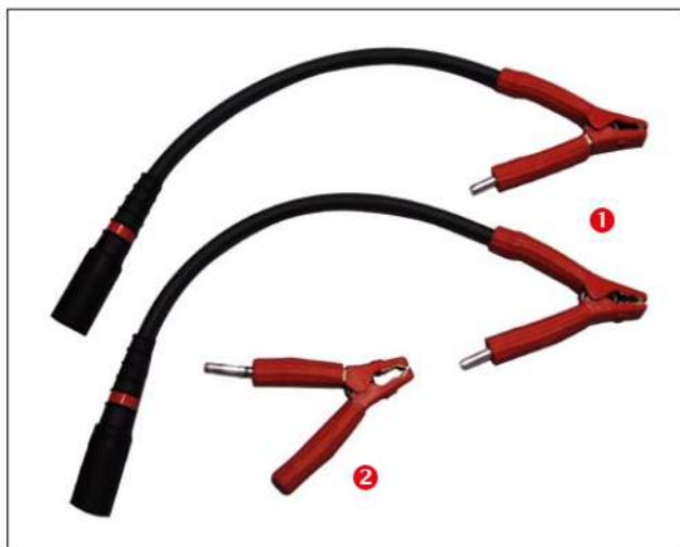
Комплект подключения СНЧ CS-BB (3-фазный)
