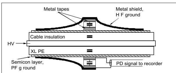
Рис. 6: Датчик, установленный в силовой кабель
