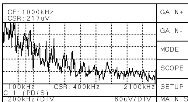
Рис. 2: Пример представления на экране спектра
