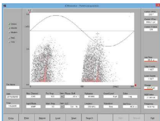
Рис. 4: Изображение на экране шаблона распределения накопленных ЧР, представленных в цвете
