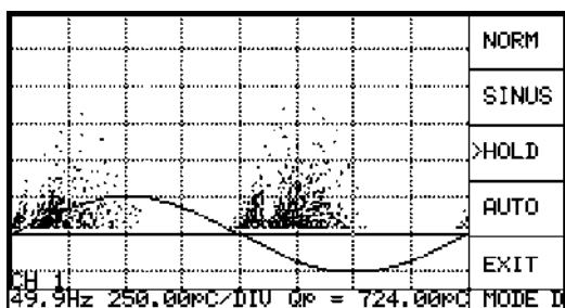
Рис. 1: Монохромное изображение ЧР (осциллографический режим)
