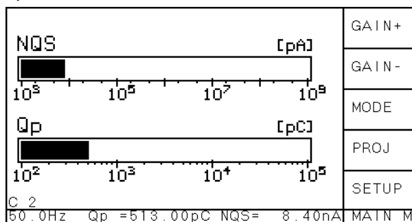
Рис. 3: Экран дисплея для режима проекционного отображения (в столбце справа регулировки коэффициента усиления, выбор режима работы, настройки и т.д.)
