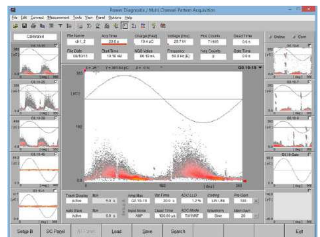
Рис. 10: Мультиплексный сбор образцов ЧР
