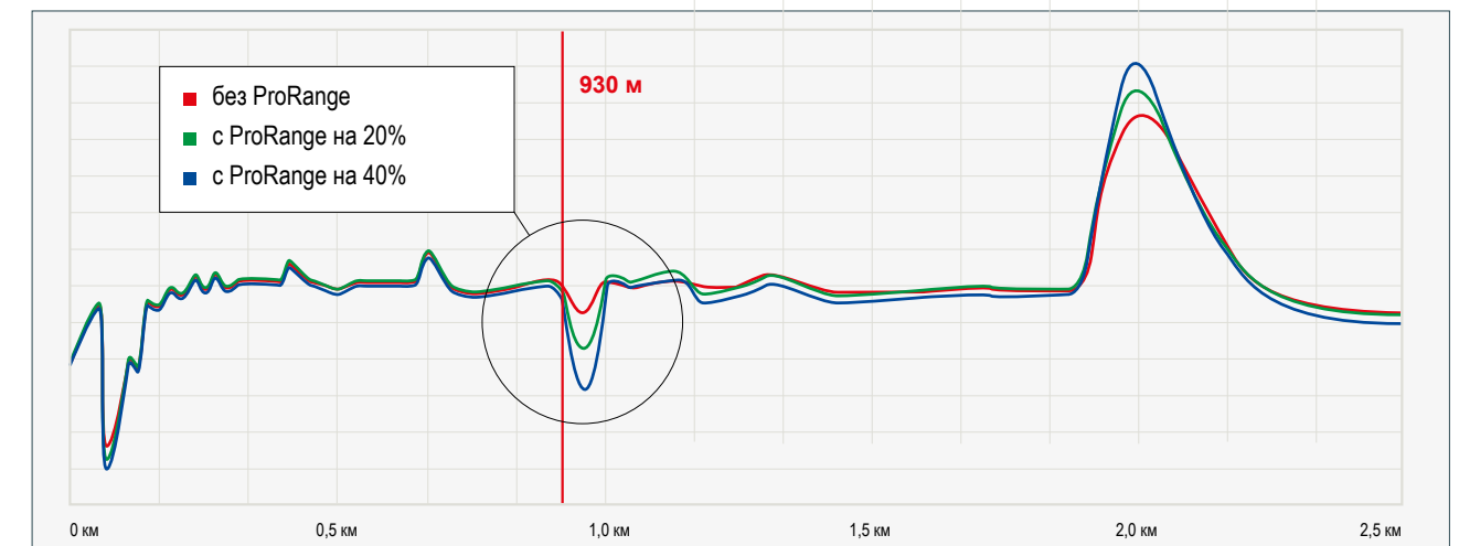
ProRange – компенсация затухания в зависимости от расстояния
